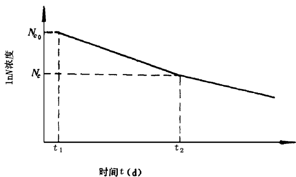
地区综合求 k_c 图解法
